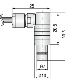
Connecteur type B/90
