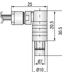
Stecker Typ B/90
