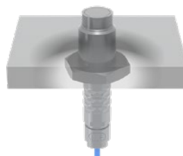
後ろ側からナットで固定
