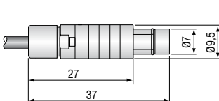
Stecker Typ B
