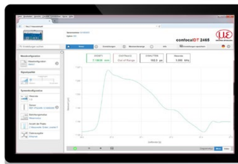
Tutte le impostazioni vengono eseguite tramite l'interfaccia web. Per la misurazione dello spessore è presente un database dei materiali che può essere ampliato a piacimento.
