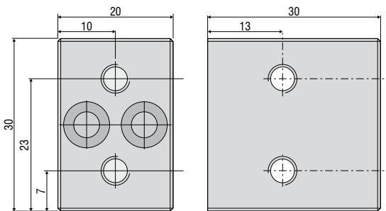
마운팅 블록
