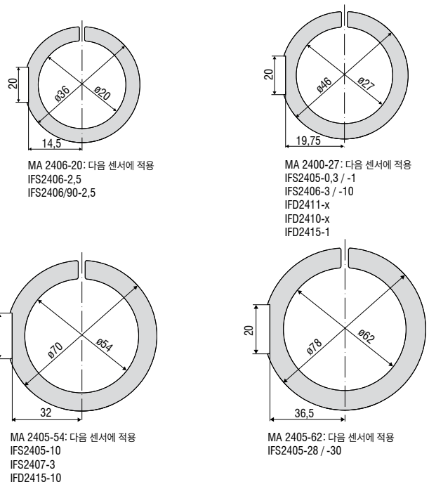
마운팅 링
