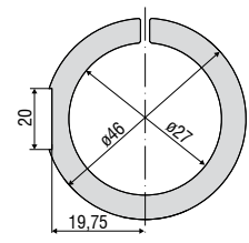
MA 2400-27: 다음 센서에 적용 IFS2405-0,3 / -1 IFS2406-3 / -10 IFD2411-x IFD2410-x IFD2415-1
