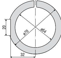
MA 2405-54: 다음 센서에 적용 IFS2405-10 IFS2407-3 IFD2415-10
