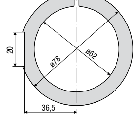
MA 2405-62: 다음 센서에 적용 IFS2405-28 / -30
