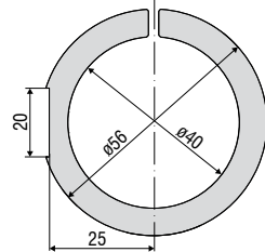
MA 2405-40: 다음 센서에 적용 IFS2405-6
