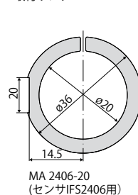
取付リング
