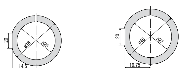
마운팅 링
