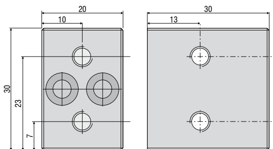
마운팅 블록
