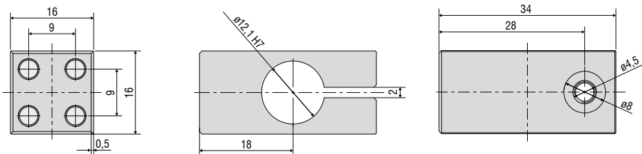
Zubehör: Sensor-Montageadapter MA2404-12 für Sensoren IFS2404-2 / IFS2404/90-2 / IFS2407-0,1
