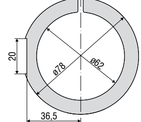
MA 2405-62 pour capteurs IFS2405-28 / -30
