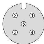
Connettore a 5 poli M12x1 Vista lato pin
