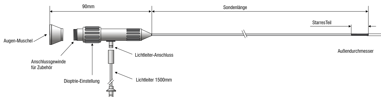
Lötstellen prüfen
