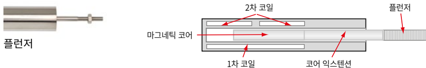
측정 원리: 변위센서
