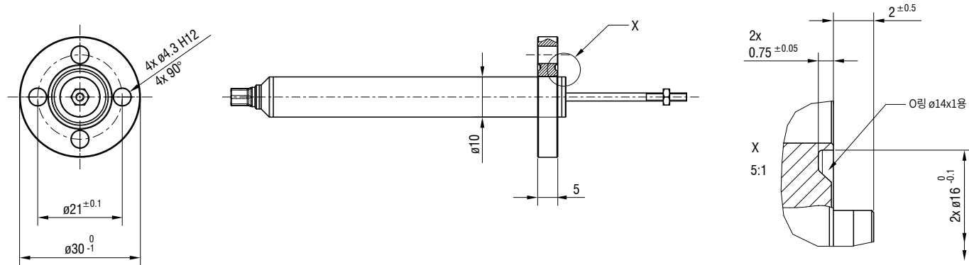
DTA-1DX, 3DX, 5DX, 10DX 가압 플랜지
