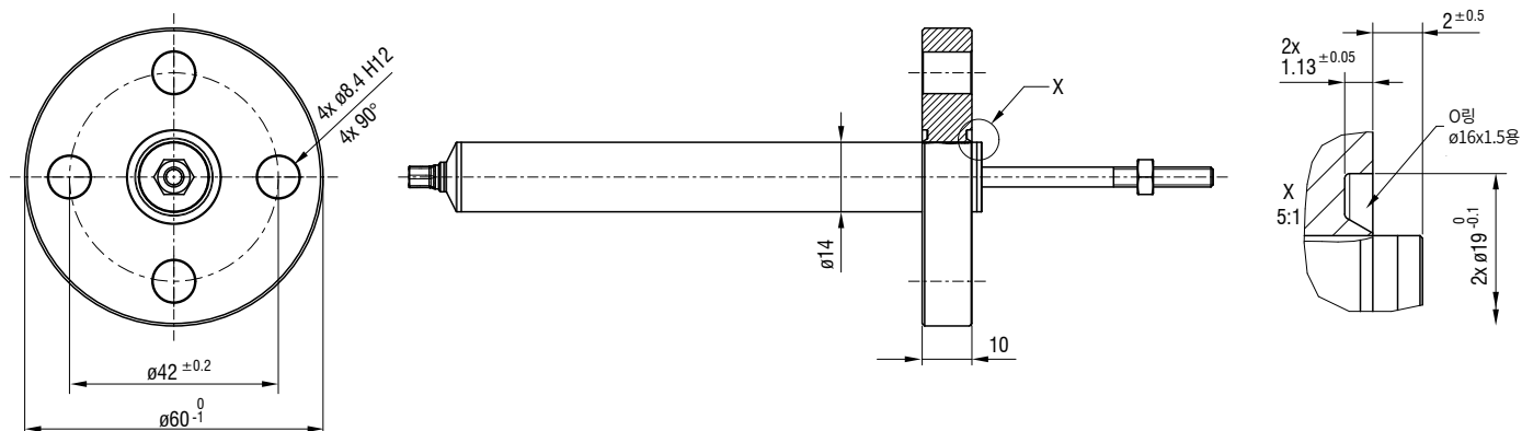
DTA-15DX, 25DX 가압 플랜지
