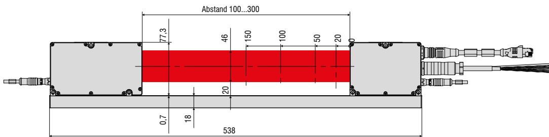
Lichtquelle und Empfänger mit Montageschiene
