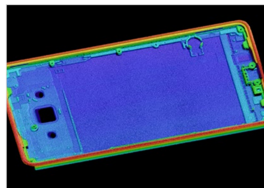
Nuage de points 3D de la plaque de support du smartphone dans 3DInspect
