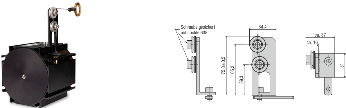
TR5-WDS(04) Integrierte Doppelumlenkrolle, 90° abgewinkelt, für Baureihe P115 mit Seildurchmesser 0,45 mm
