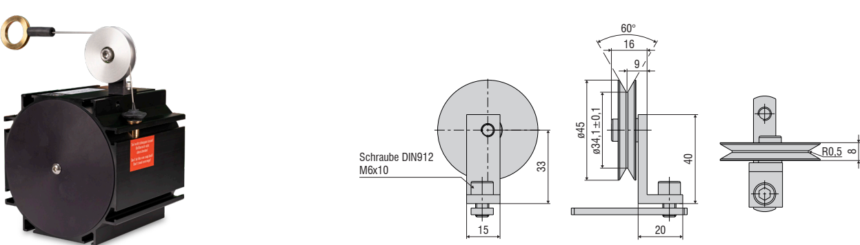
TR6-WDS(01) Integrierte Seilumlenkrolle für Baureihe P115 mit Seildurchmesser 1 mm
