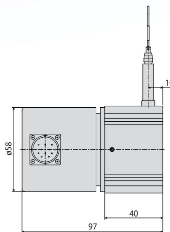
出力 SSI
