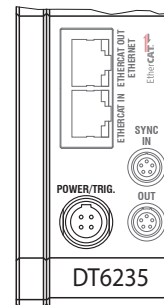
Versorgungseingang am Controller, 4-pol. Stecker
