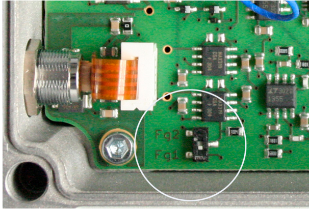
Abb. 13 Schalter Grenzfrequenz auf dem Demodulatoremodul
