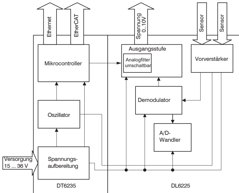
Abb. 2 Blockschaltbild capaNCDT 6235
