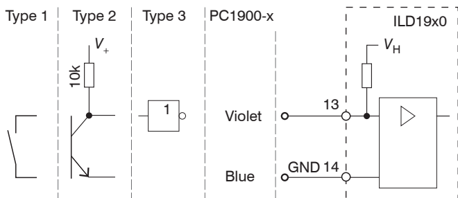
Fig. 22 Circuit schématique pour les entrées multifonction
