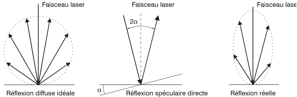
Fig. 8 Réflectivité de la surface de mesure
