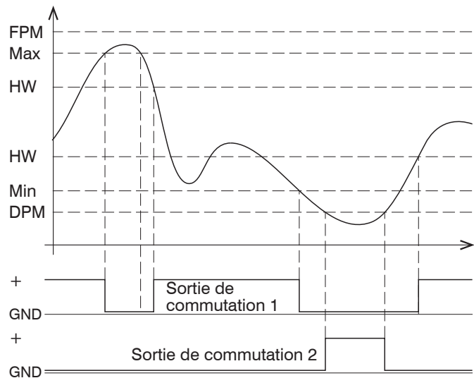
Fig. 51 Sortie de commutation 1 avec valeurs limites (NPN), sortie de commutation 2 avec erreur de plage de mesure (PNP)
