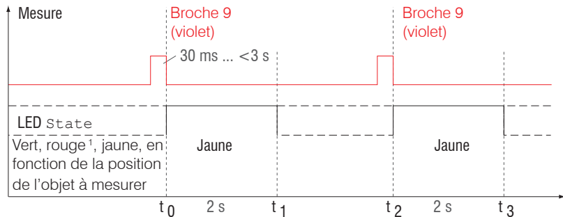
Fig. 42 Organigramme pour la remise à zéro et l'étalonnage (entrée matérielle)
