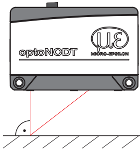
Fig. 12 Montage du capteur en cas de réflexion diffuse
