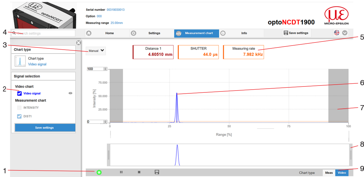
Fig. 30 Site Web du signal vidéo
