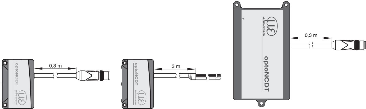
ILD1900 avec pigtail
