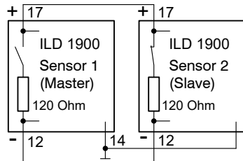
Fig. 33 Le capteur 1 synchronise un autre capteur
