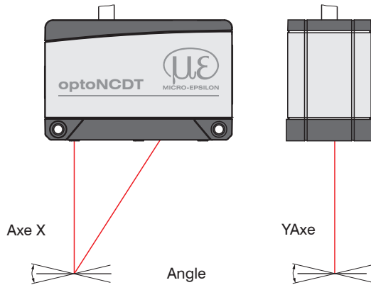
Fig. 9 Erreurs de mesure dues à l'inclinaison en réflexion diffuse
