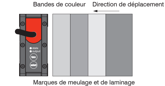
Fig. 10 Agencement du capteur pour les surfaces meulées ou striées
