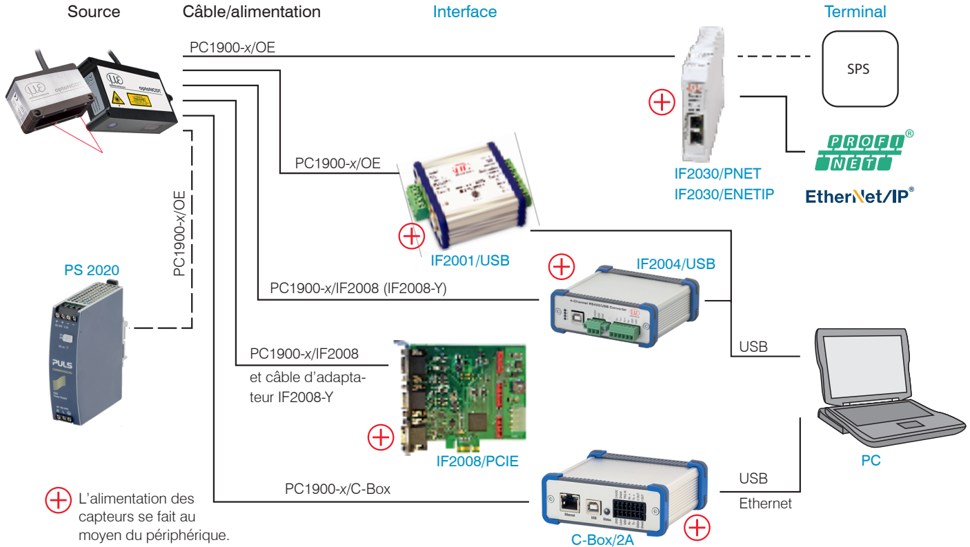
Fig. 17 Exemples de branchement sur l'ILD1900
