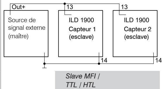
Fig. 35 Synchronisation des capteurs par la source de signal
