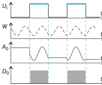
Fig. 37 Niveau de déclenchement haut (supérieur) avec sortie analogique A_0 et signal de sortie numérique D_0 (inférieur)
