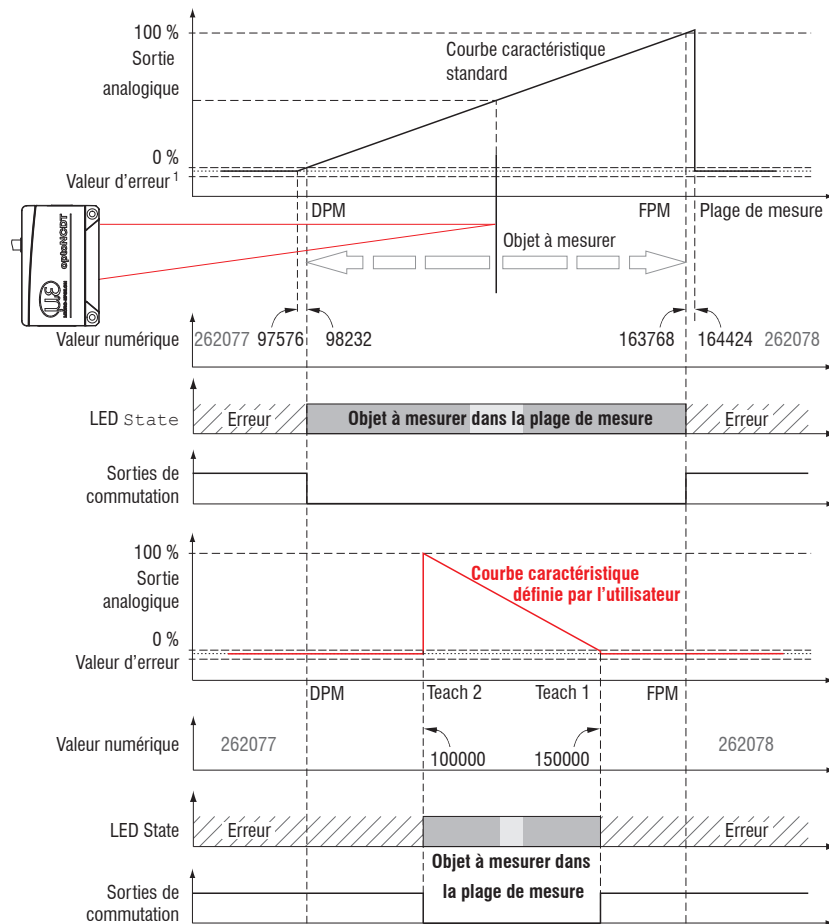
1) Avec sortie de courant 3,0 mA.
