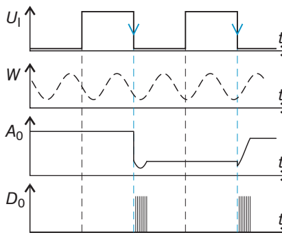
Fig. 38 Flanc de déclenchement HL (supérieur) avec sortie analogique A_0 et signal de sortie numérique D_0 (inférieur)
