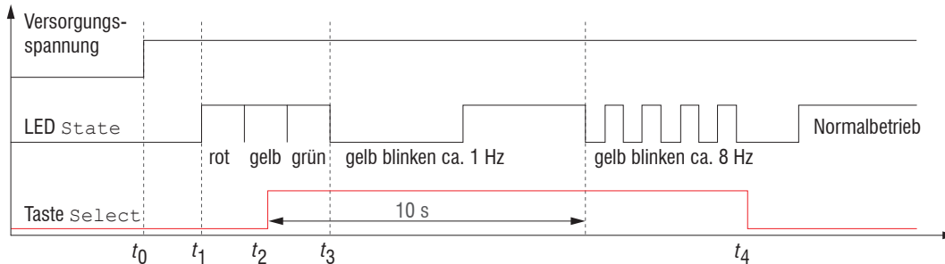
Fig. 57 Organigramme de démarrage d'un capteur avec les paramètres d'usine
