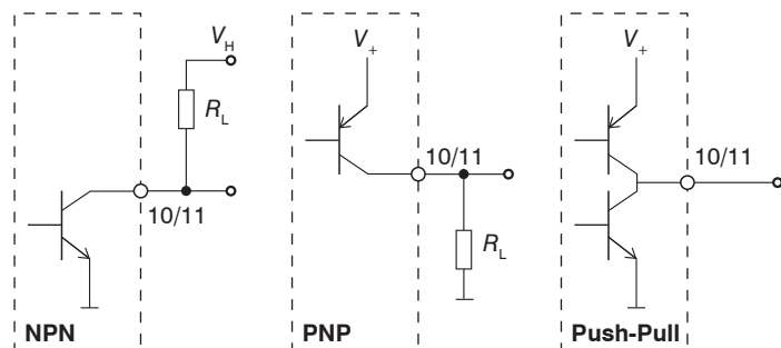
Fig. 24 Circuit schématique de la sortie de commutation
