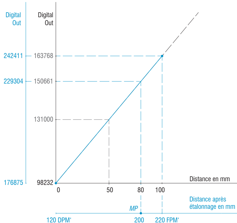
Fig. 45 Valeurs numériques ILD1900-100 après étalonnage avec valeur étalon de 200 mm
