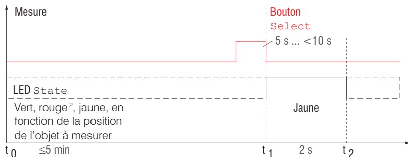
Fig. 41 Organigramme d'annulation de l'opération de remise à zéro / étalonnage
