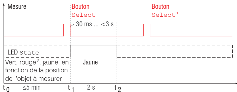
Fig. 40 Organigramme pour la remise à zéro et l'étalonnage (bouton Select)
