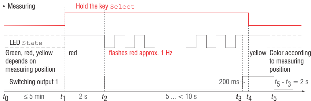
Fig. 48 Organigramme de réinitialisation de la mise à l'échelle des sorties
