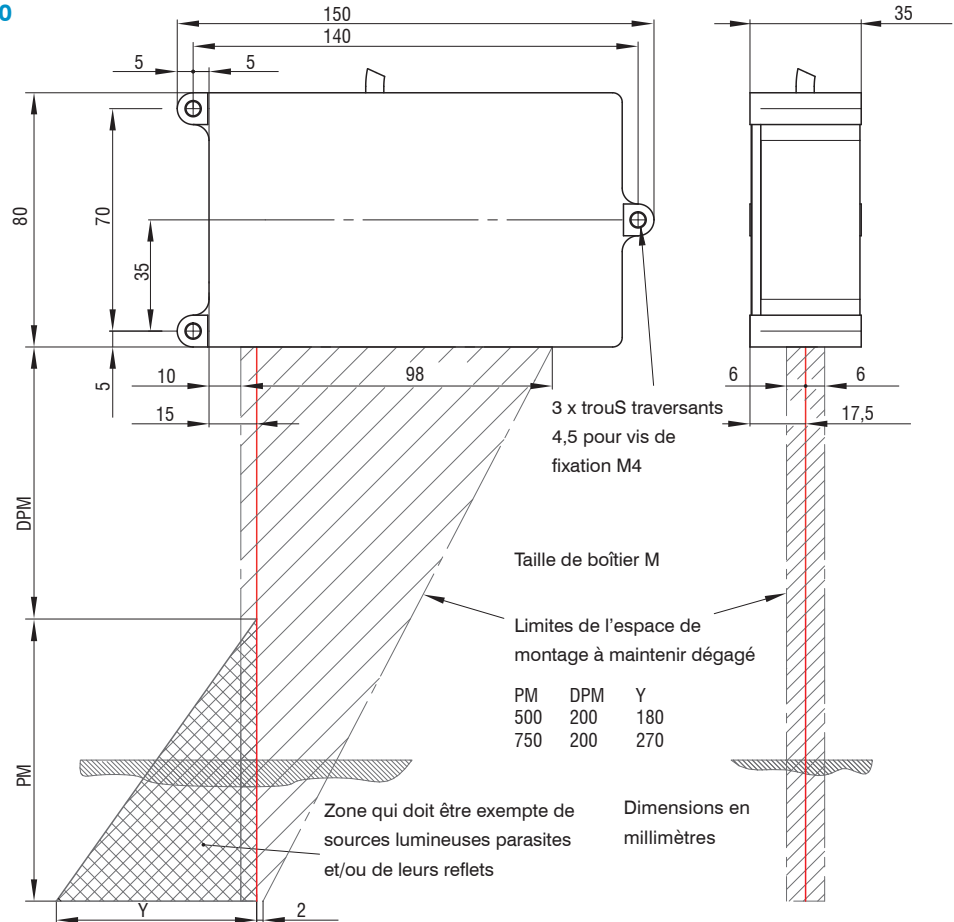
Fig. 16 Dessin coté et dégagement, ILD1910-500/750
