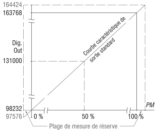
Fig. 44 Valeurs numériques sans remise à zéro ni étalonnage (mastering)
