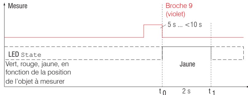
Fig. 43 Organigramme d'annulation de l'opération de remise à zéro / étalonnage
