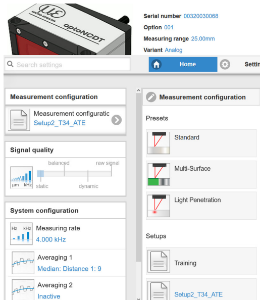
Fig. 28 Extrait de l'interface web, onglet Home
