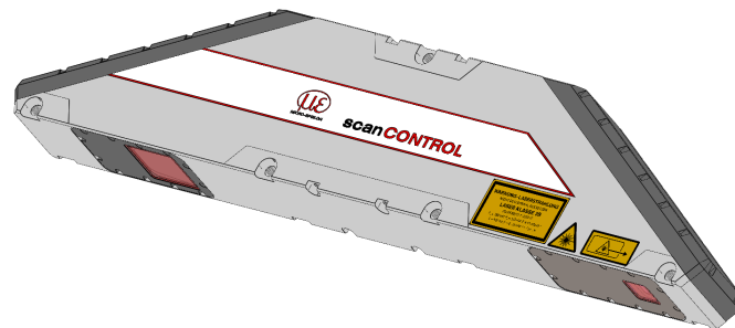
Abb. 2 Sensor mit offenem Strahlfänger
