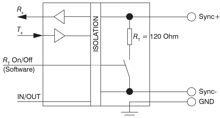
Abb. 24 Innenschaltung Synchronisation RS422
