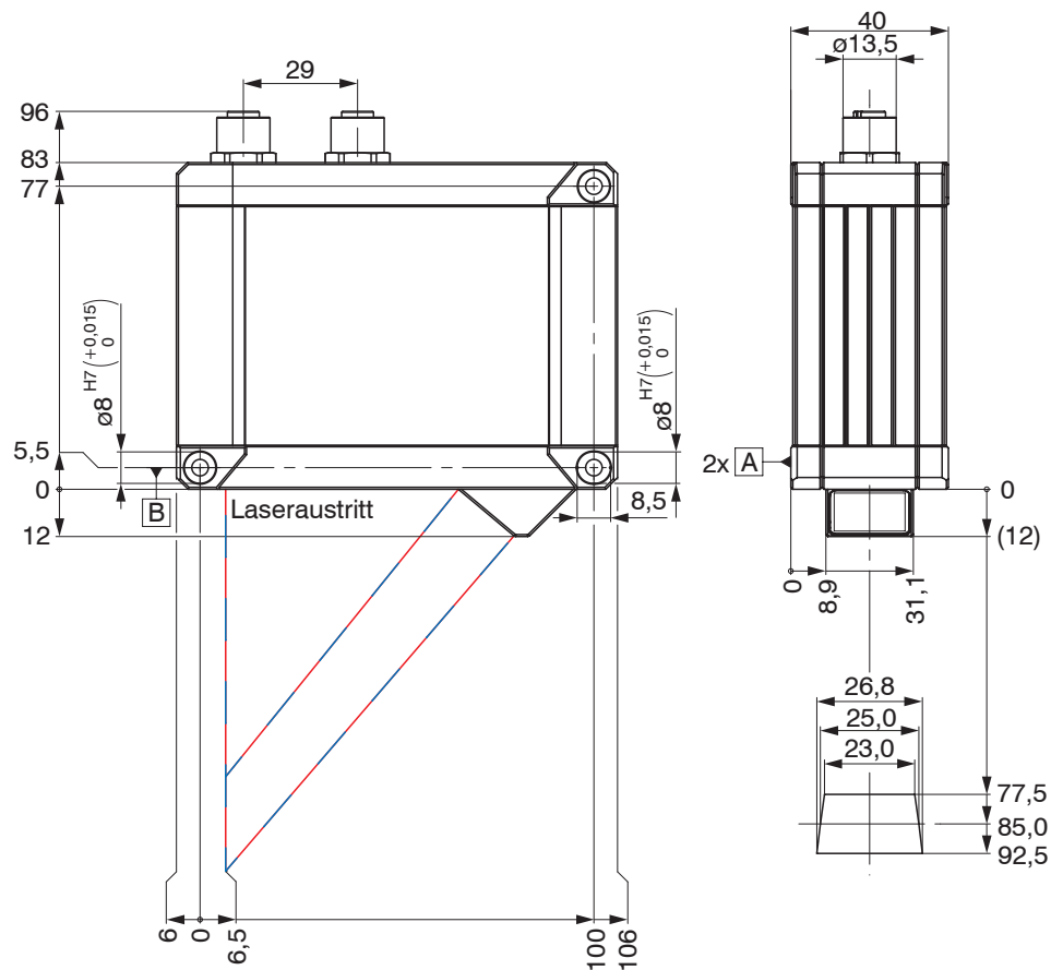
Abb. 15 Maßzeichnung Sensor scanCONTROL 30xx-25, Abmessungen in mm
