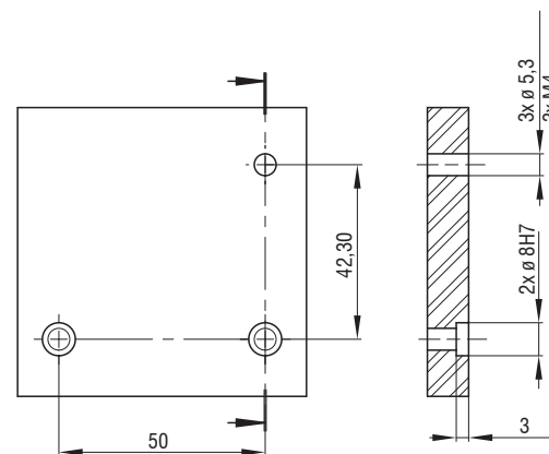
Abb. 10 Maßzeichnung Montagebohrungen, Abmessungen in mm
