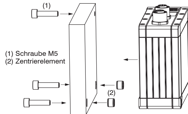
Abb. 5 Montagebeispiel direktes Anschrauben
