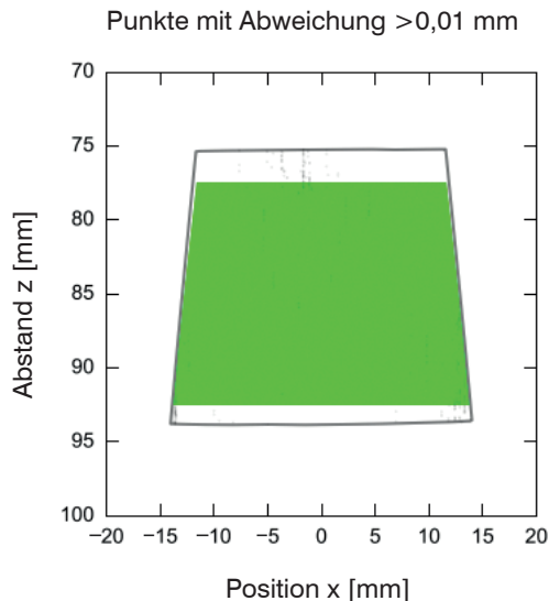
Abb. 32 Linearitätsabweichung, Beispiel eines scanCONTROL 30xx-25
