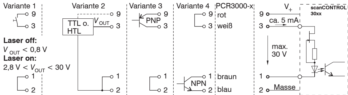
Abb. 29 Möglichkeiten für die externe Laserabschaltung
