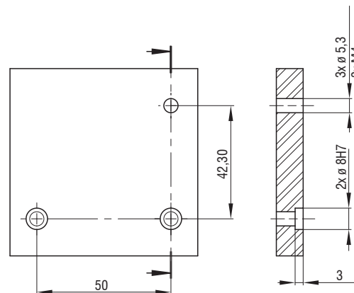
Abb. 8 Maßzeichnung Montagebohrungen, Abmessungen in mm
