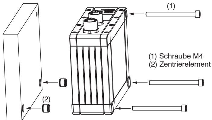
Abb. 4 Montagebeispiel Durchsteckverschraubung
