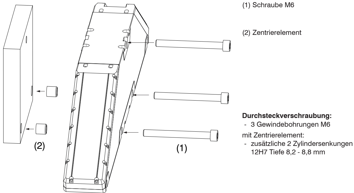
Abb. 12 Montagebeispiel Durchsteckverschraubung LLT30xx-430 / LLT30xx-600
