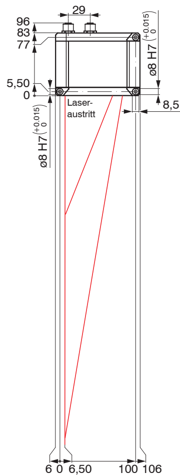
Abb. 18 Maßzeichnung Sensor scanCONTROL 30xx-200, Abmessungen in mm
