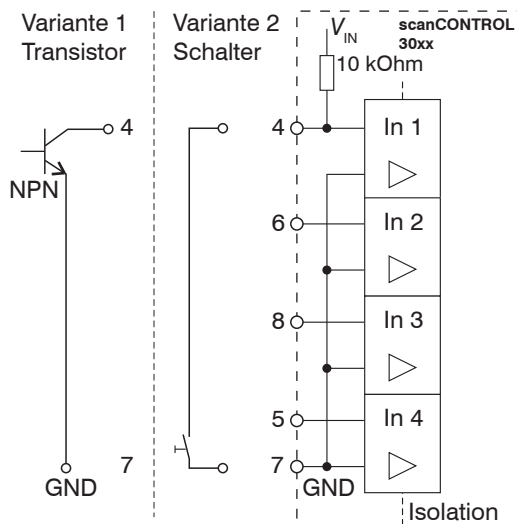
Abb. 26 Pull-up
