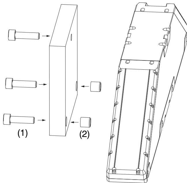
Abb. 11 Montagebeispiel direktes Anschrauben LLT30xx-430 / LLT30xx-600
