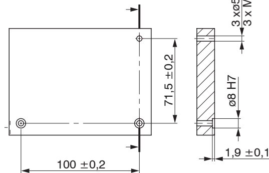
Abb. 6 Maßzeichnung Montagebohrungen, Abmessungen in mm
