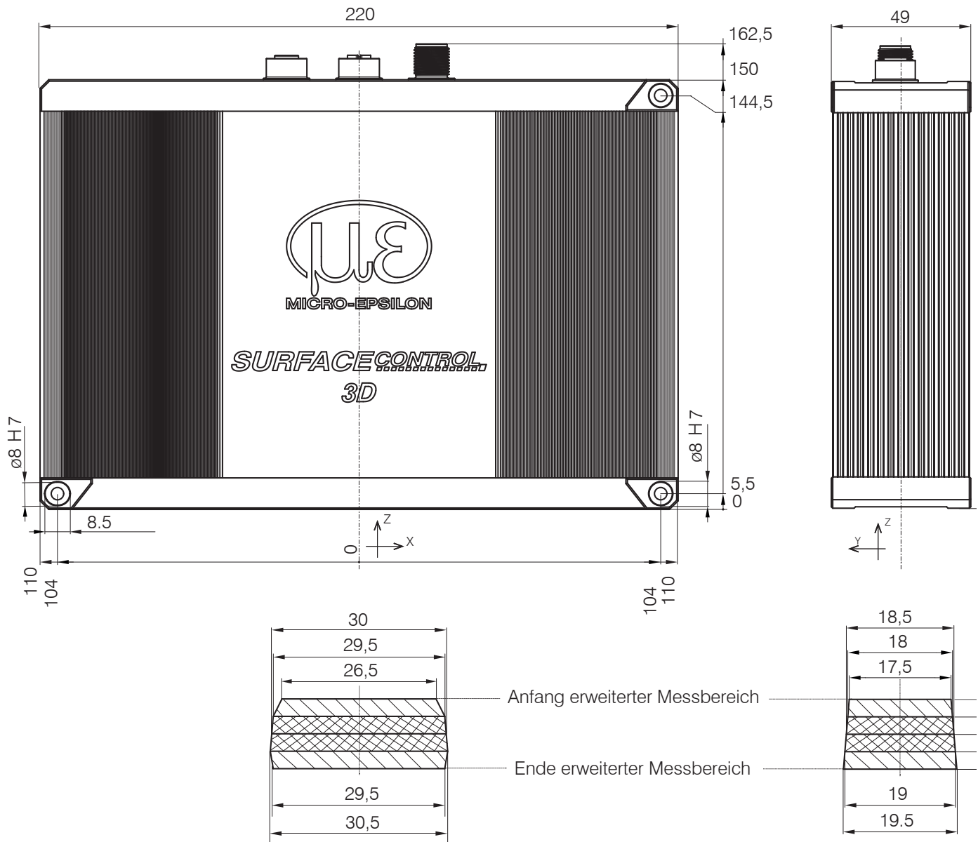
Abb. 9 Maßzeichnung Sensor surfaceCONTROL 3D 32xx-30, Abmessungen in mm
