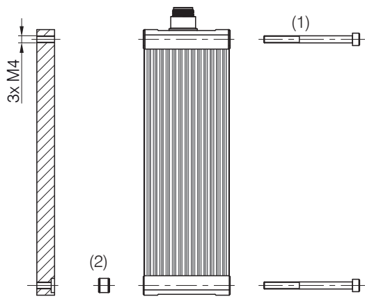
Abb. 5 Montagebeispiel Durchsteckverschraubung
