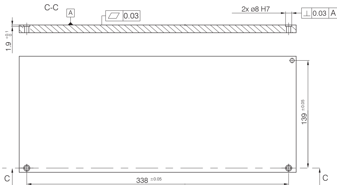
Abb. 8 Maßzeichnung Montagebohrungen, Sensor surfaceCONTROL 3D 35xx-240, Abmessungen in mm
