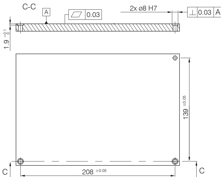
Abb. 7 Maßzeichnung Montagebohrungen, Sensor surfaceCONTROL 3D 35xx-80 und surfaceCONTROL 3D 32xx-120, Abmessungen in mm
