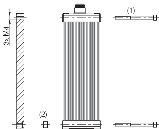
Abb. 5 Montagebeispiel Durchsteckverschraubung
