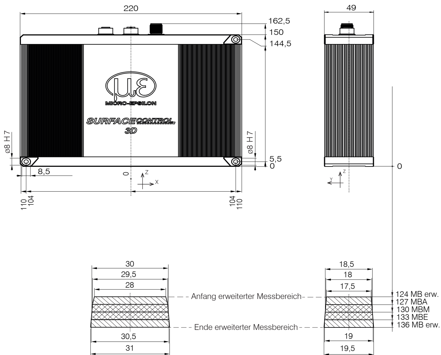
Abb. 9 Maßzeichnung Sensor surfaceCONTROL 3D 35xx-30, Abmessungen in mm
