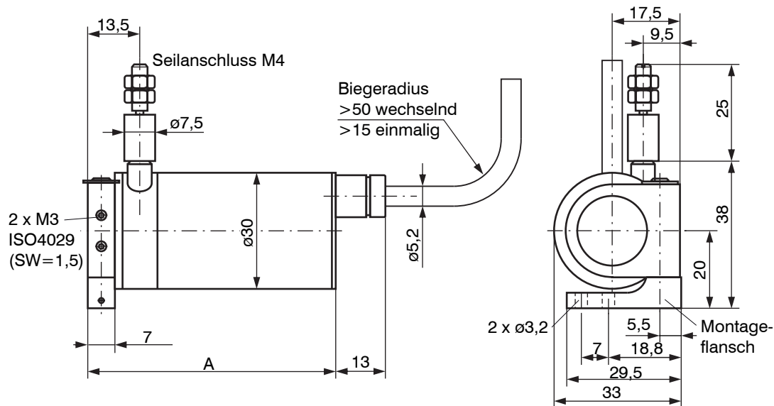
Abb. 6 Maßzeichnung Baureihe WDS - ... - MPM, Abmessungen in mm
