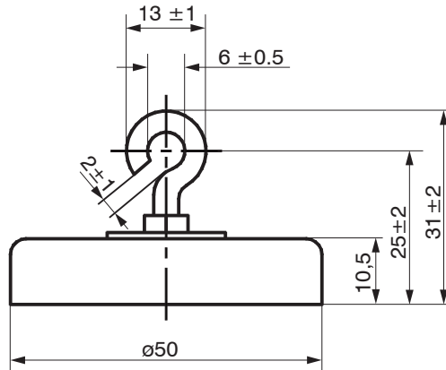
Abb. 10 Magnethalter MH1 - WDS, Abmessungen in mm
