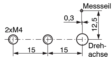
Abb. 5 Bohrbild Baureihe WDS - ... - MP / MPW, Abmessungen in mm
