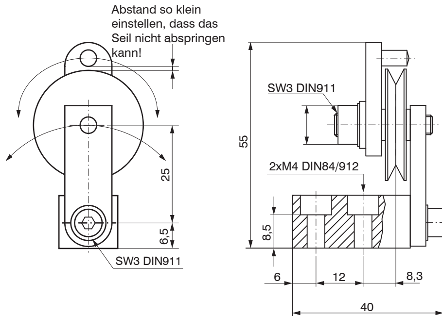
Abb. 11 Umlenkrolle TR1-WDS mit Montagefuß, Abmessungen in mm
