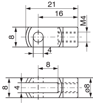
Abb. 14 Gabelkopf mit Federklappbolzen GK1-WDS, Abmessungen in mm
