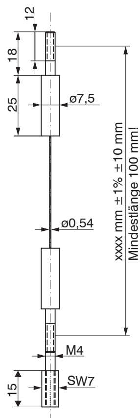
Abb. 13 Seilverlängerung WE-xxxx-M4, Abmessungen in mm
