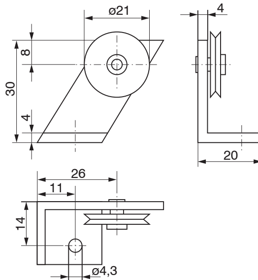
Abb. 12 Umlenkrolle TR3-WDS, fest, mit Montagefuß, Abmessungen in mm
