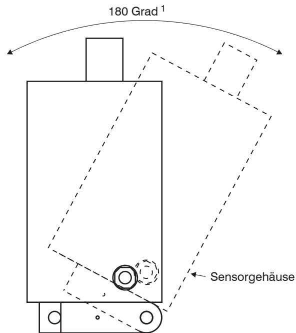
Abb. 3 Horizontale Drehung des Sensorgehäuses
