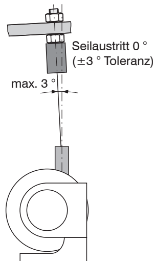
Abb. 8 Befestigung und maximaler Schrägzug des Messseils
