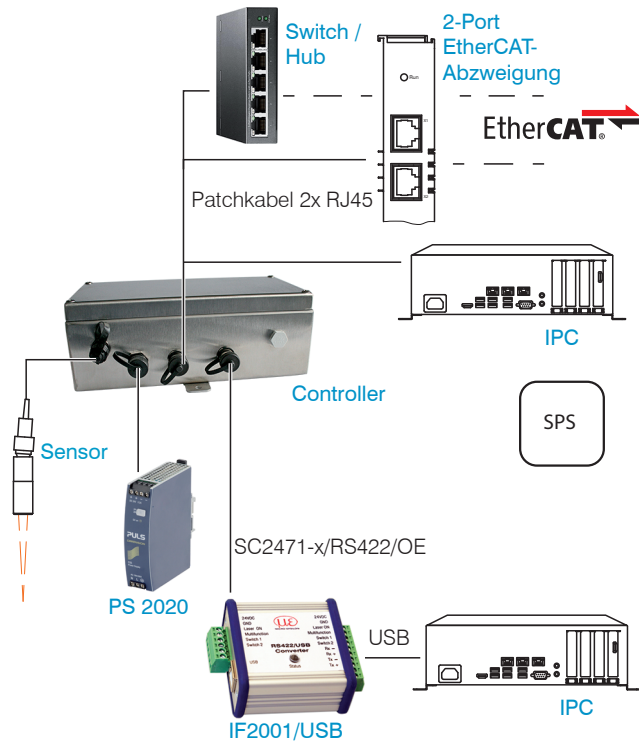
Anschlussbeispiele am IMS5420IP67, IMS5420IP67MP
