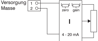
Ausführung mit Stromausgang
