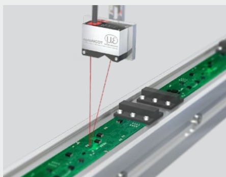
Impiego nell'assemblaggio di circuiti stampati
