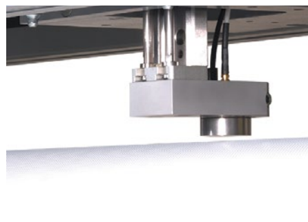
Misurazione in linea senza contatto dello spessore delle pellicole
