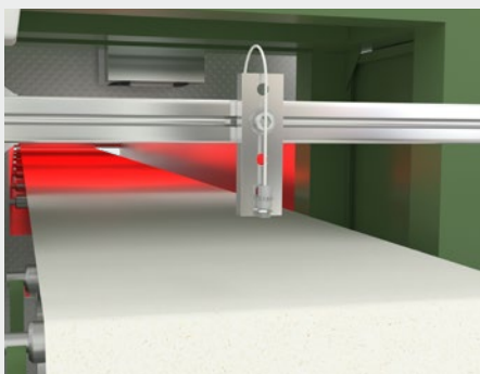
Monitoraggio del processo di essiccazione nella produzione di carta
