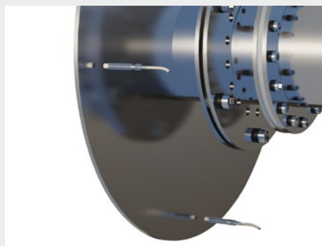
Misurazione del gioco radiale dei dischi della frizione
