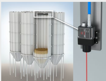
連続した充填レベル測定
