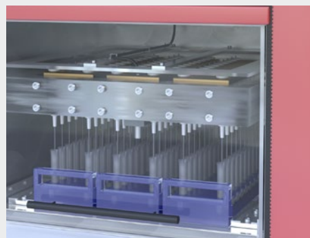
DNA分析装置内の試料の温度測定
