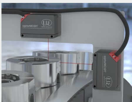
旋盤加工部品の寸法検査
