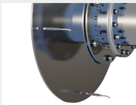
Mesure de l'impact radial des disques d'embrayage
