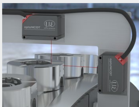
Contrôle dimensionnel des pièces pivotantes
