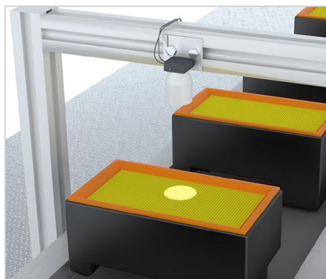
OT3シリーズのTrue Colorセンサは、測定対象物との測定距離を大きく保たなければならない測定タスク用に設計されています。
