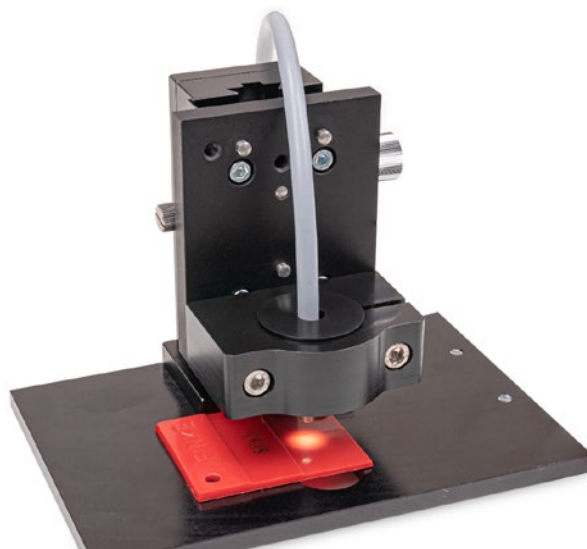
CFS4センサは、プラスチックや金属などの多種多様な表面の測色に適しています。
