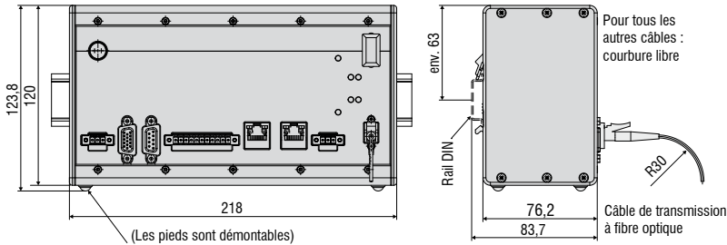
Contrôleur IFC2421
