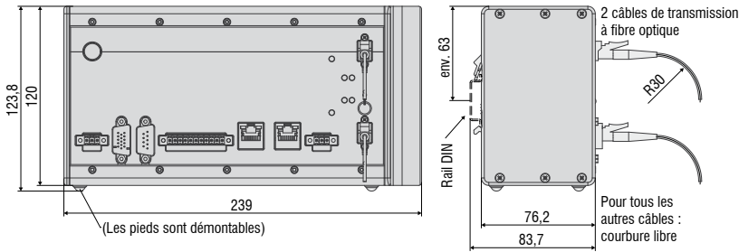
Contrôleur IFC2422
