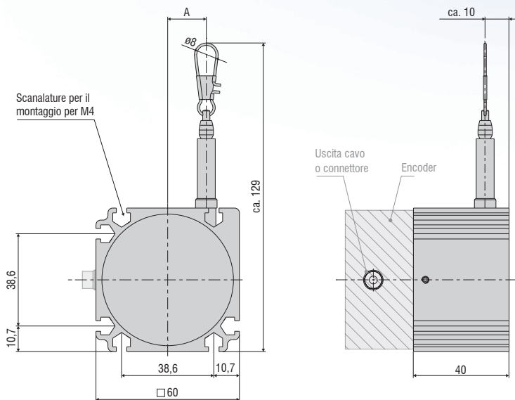
Uscita HTL/TTL
