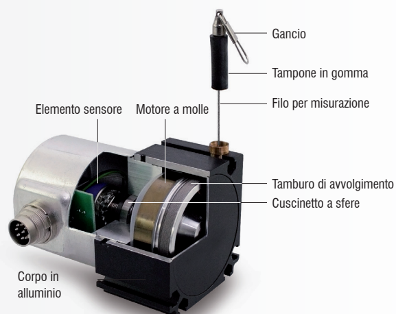
Struttura dei sensori nell'esempio del WDS-P60
