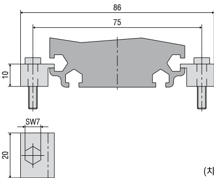
MT-60-WDS WDS-P60용 마운팅 클램프
