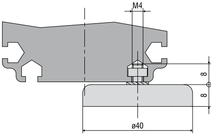
MH2-WDS 센서 설치용 마그넷 홀더
