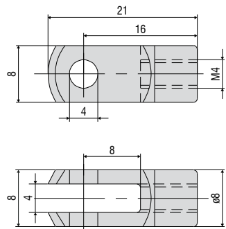
GK1-WDS M4 규격용 포크형 헤드
