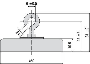
MH1-WDS 와이어 설치용 마그넷 홀더
